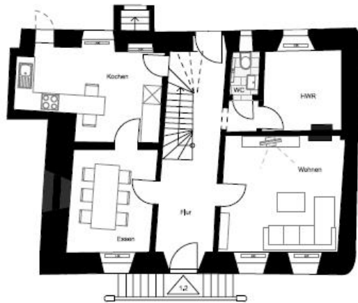
Erdgeschoss
