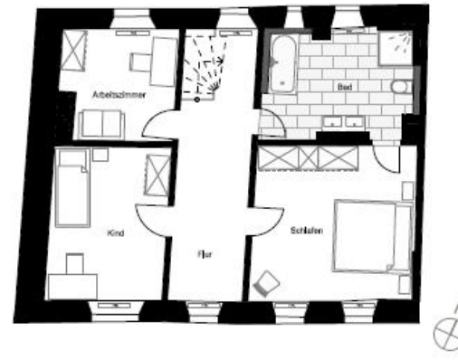
1. Obergeschoss
